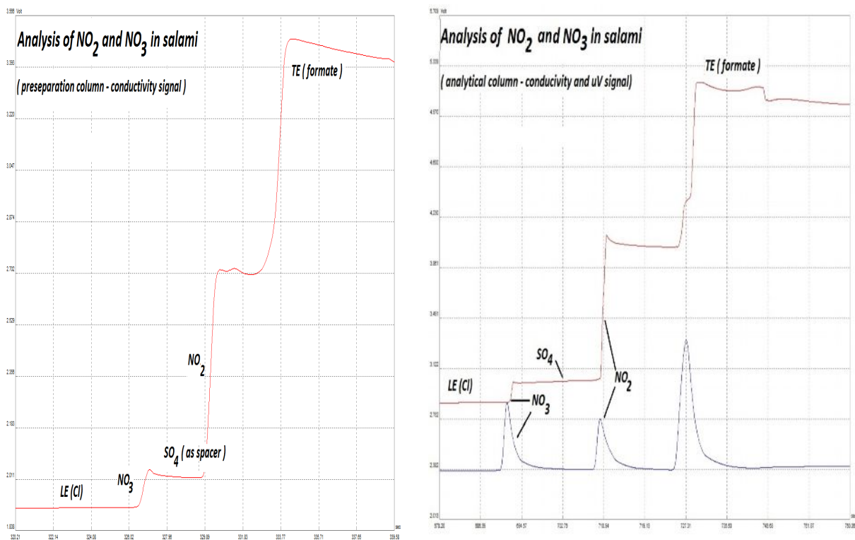
Obr.. 1: Záznam analýzy salámy v predseparačnej a analytickej kolóne
