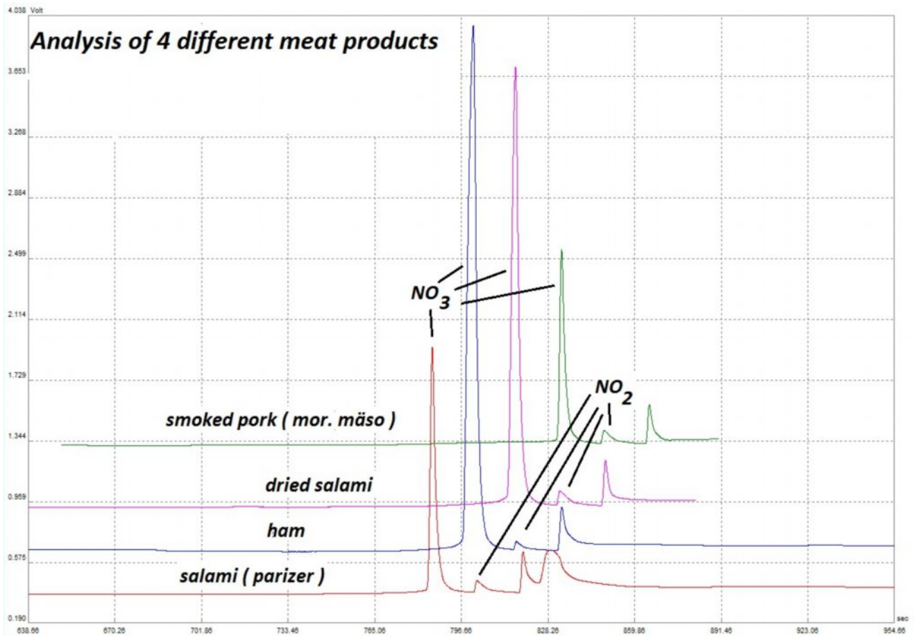
Obr. 2 : Analýza dusičnanov a dusitanov v 4 rôznych výrobkoch Podmienky ako obr.1
